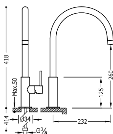
Monomando fregadero vertical MAX-TRES
