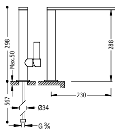
Monomando fregadero vertical CLASS-TRES caño de 34x9 mm.
